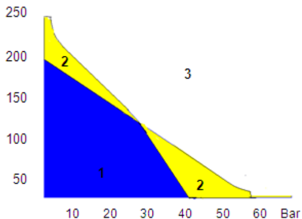
DIAGRAMA PRESION-TEMPERATURA
